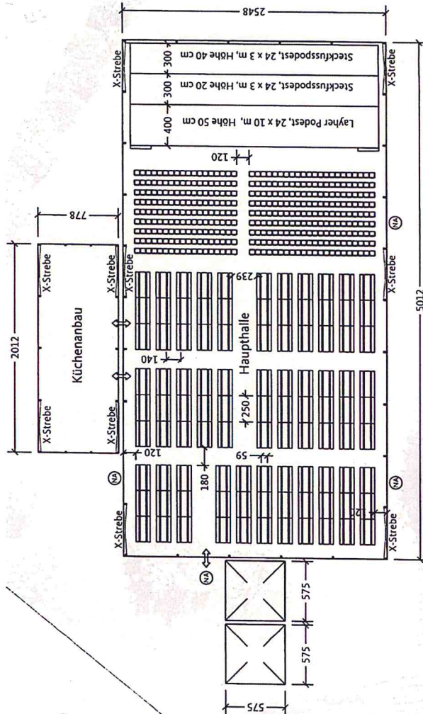
Grundriss Mst. 1:350
